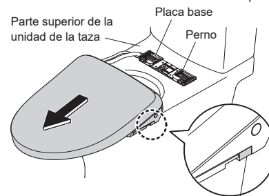
Botón de extracción de la unidad principal
